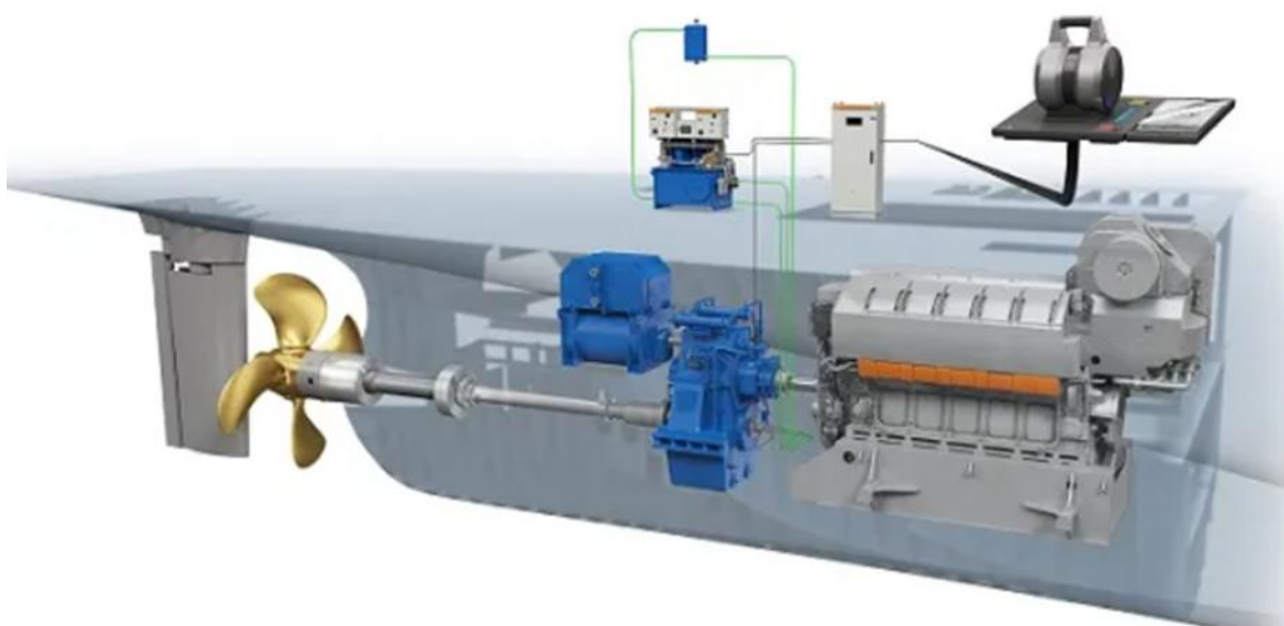
Figura 16 - Sistema de hélice acionado pelo motor do navio [28]
