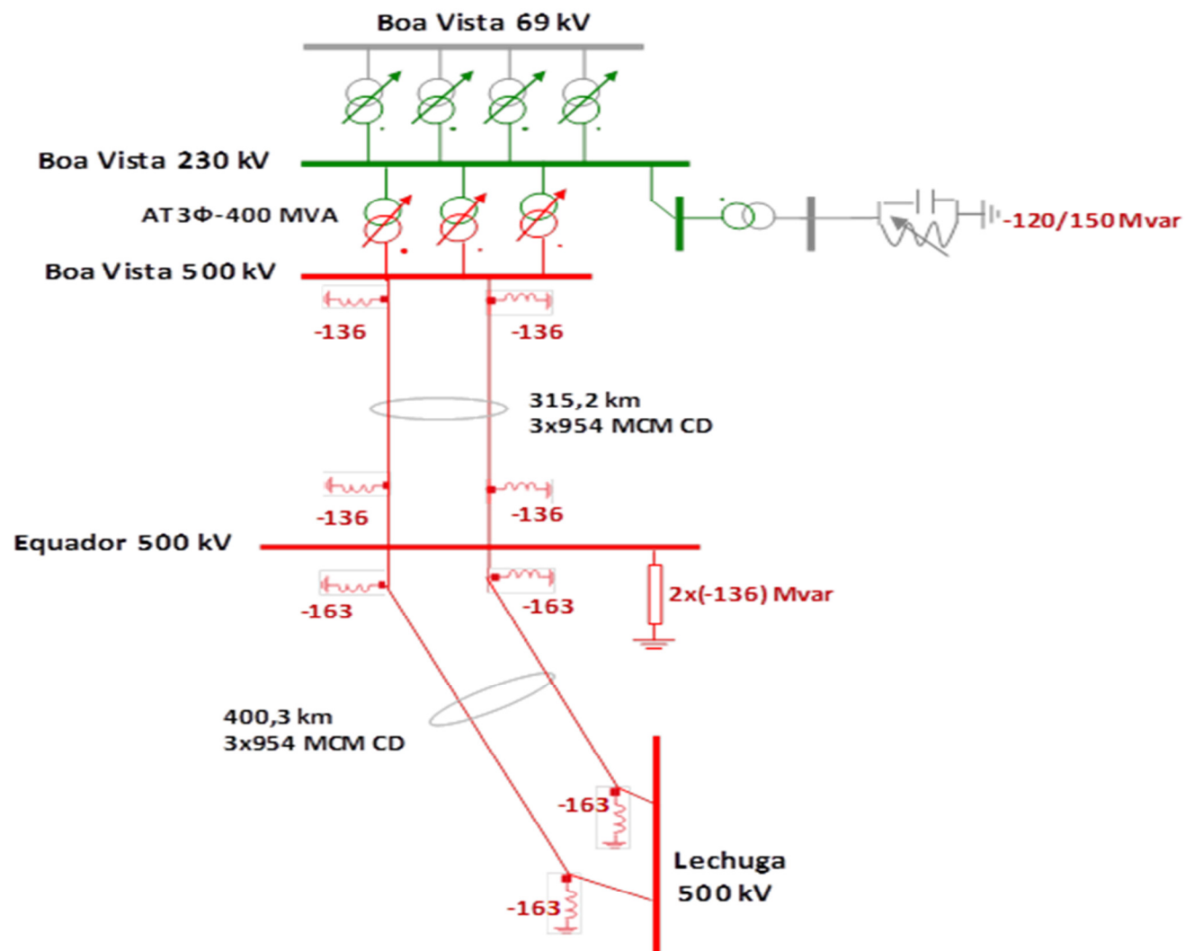
Figura 18. Interligação Manaus - Boa Vista – Unifilar
