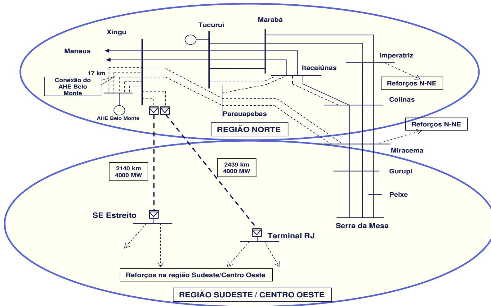
Figura 10. Reforços na interligação Norte-Sudeste/Centro-Oeste
