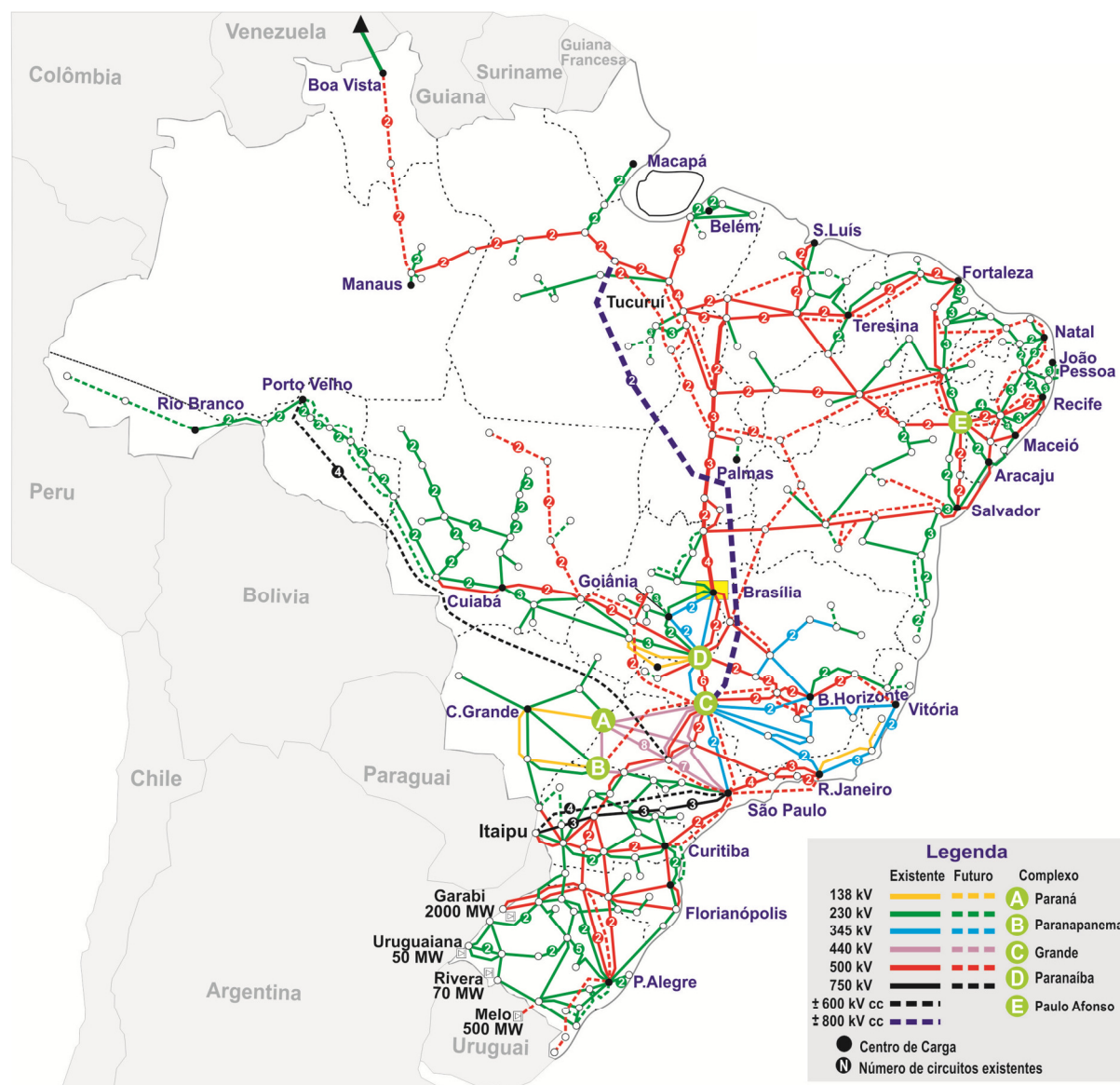
Figura 3. Diagrama do Sistema Interligado Nacional – SIN
