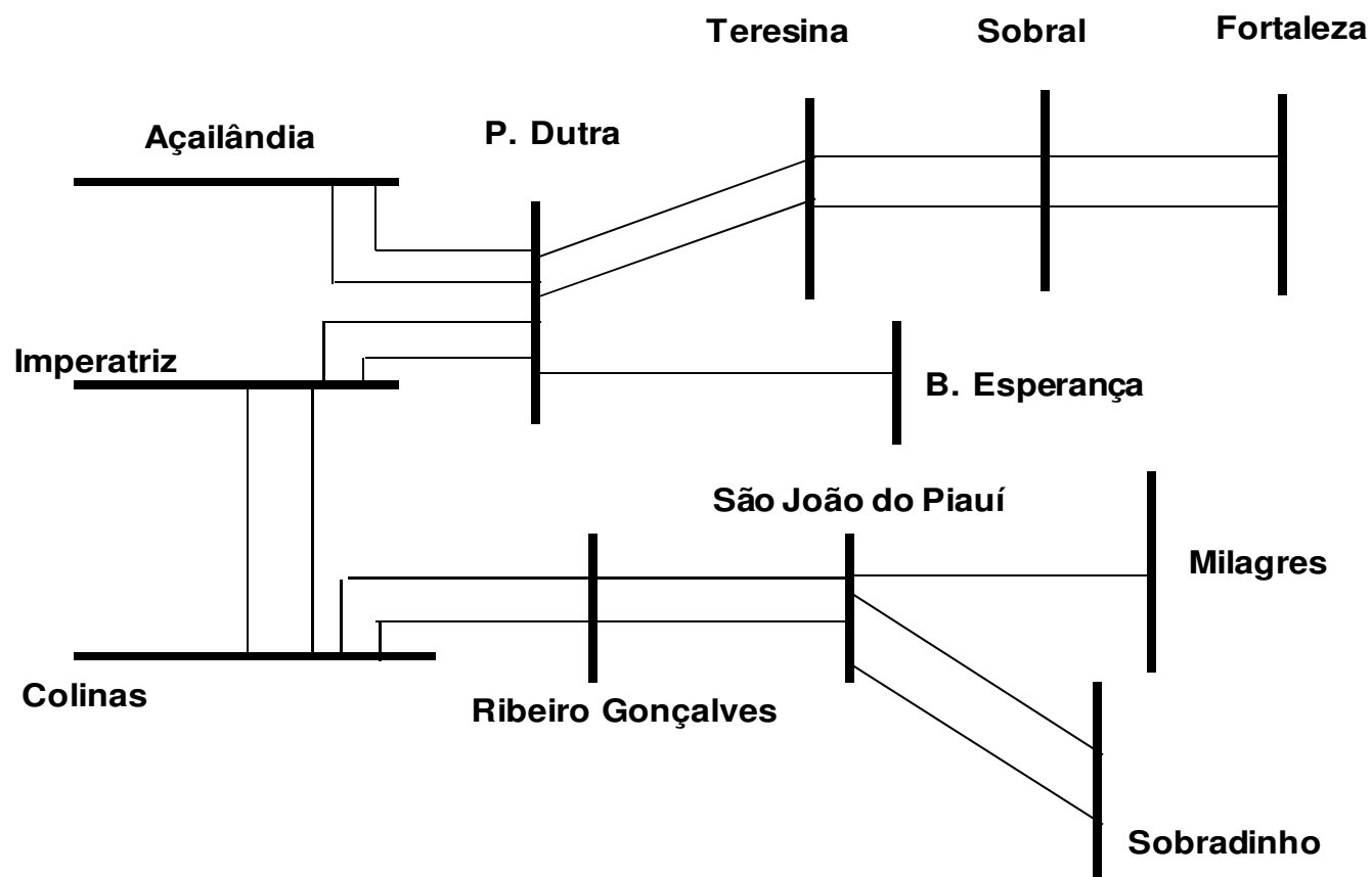
Figura 11. Diagrama esquemático da interligação Norte – Nordeste – 2017
