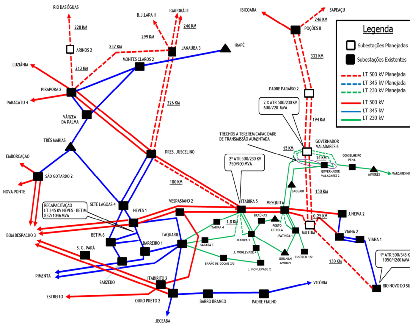
Figura 15. Expansão da Interligação Nordeste – Sudeste/Centro-Oeste
