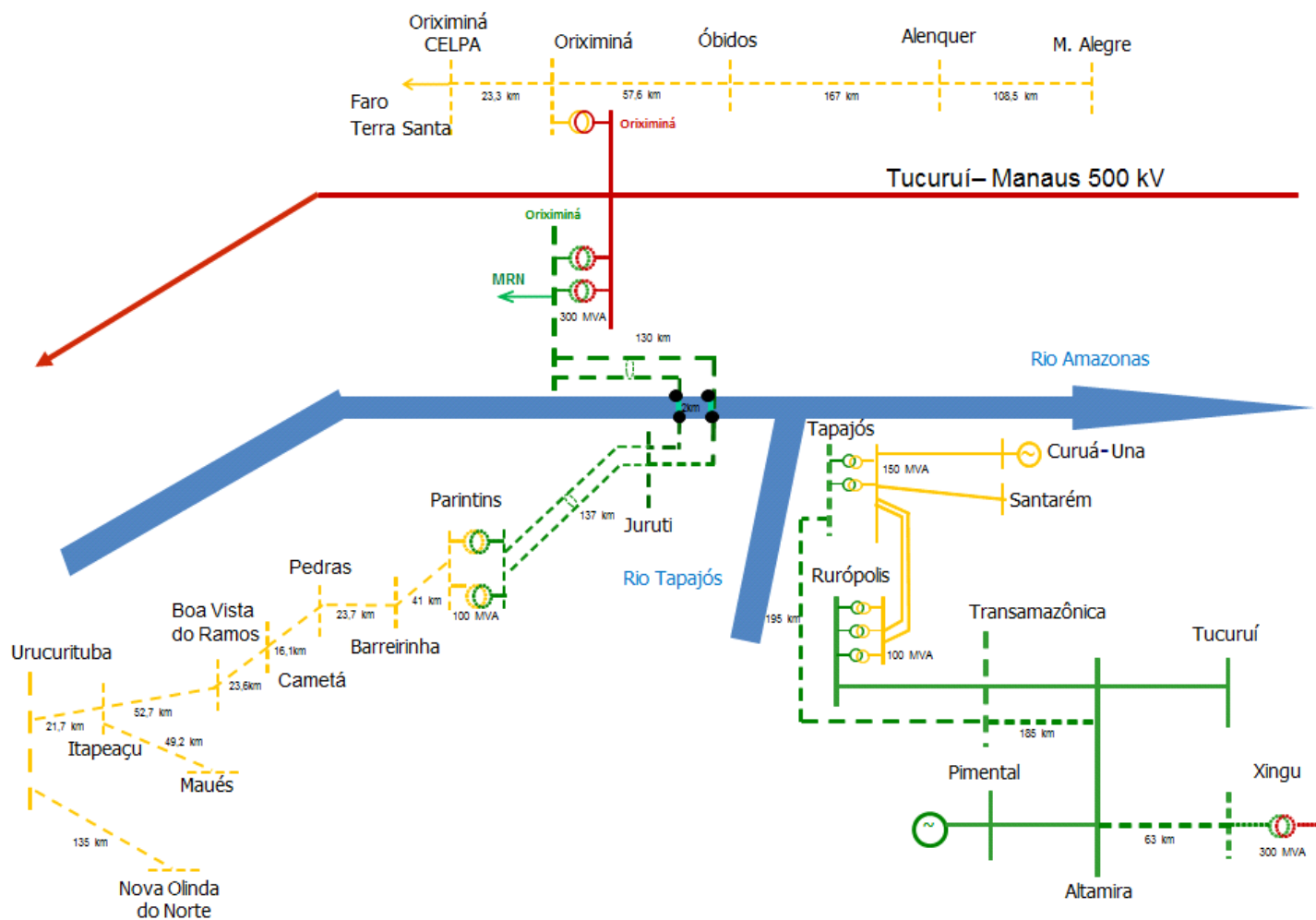
Figura 20. Interligação Oriximiná - Juruti – Parintins
