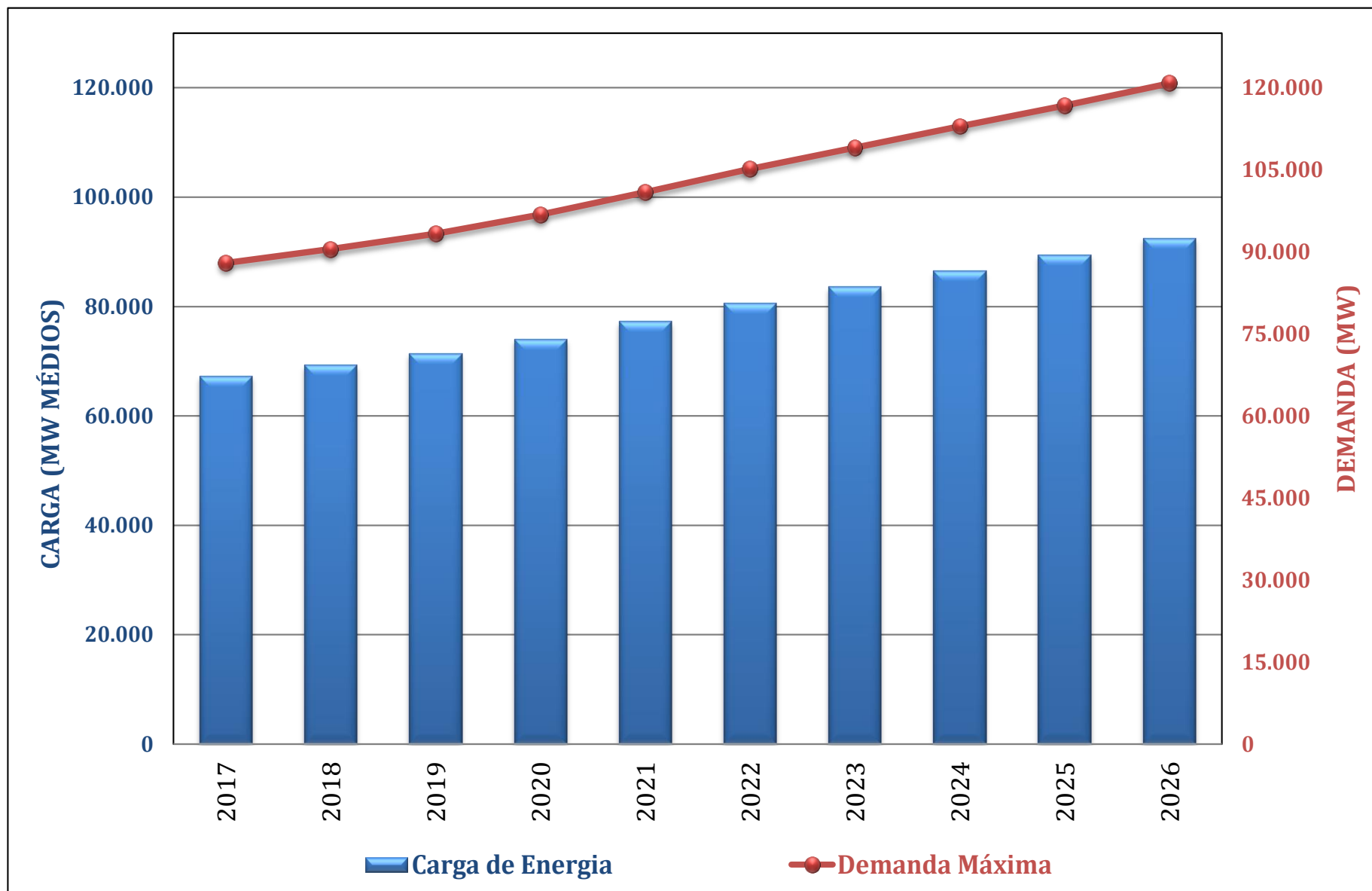
Gráfico 25. Projeção de Carga
