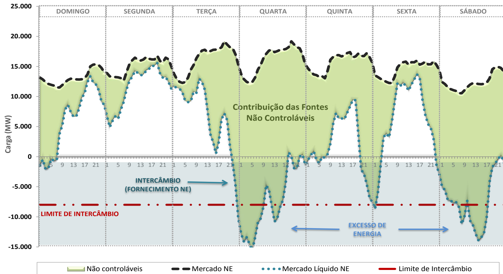
Gráfico 37. Geração das Fontes Não Controláveis - NE
