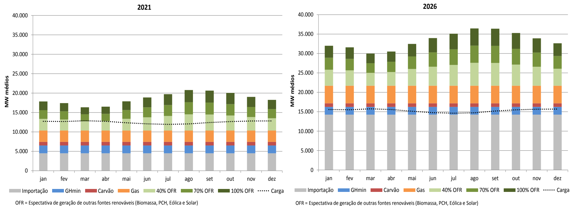
Gráfico 45. Disponibilidade de Fontes para o Atendimento da Região Nordeste
