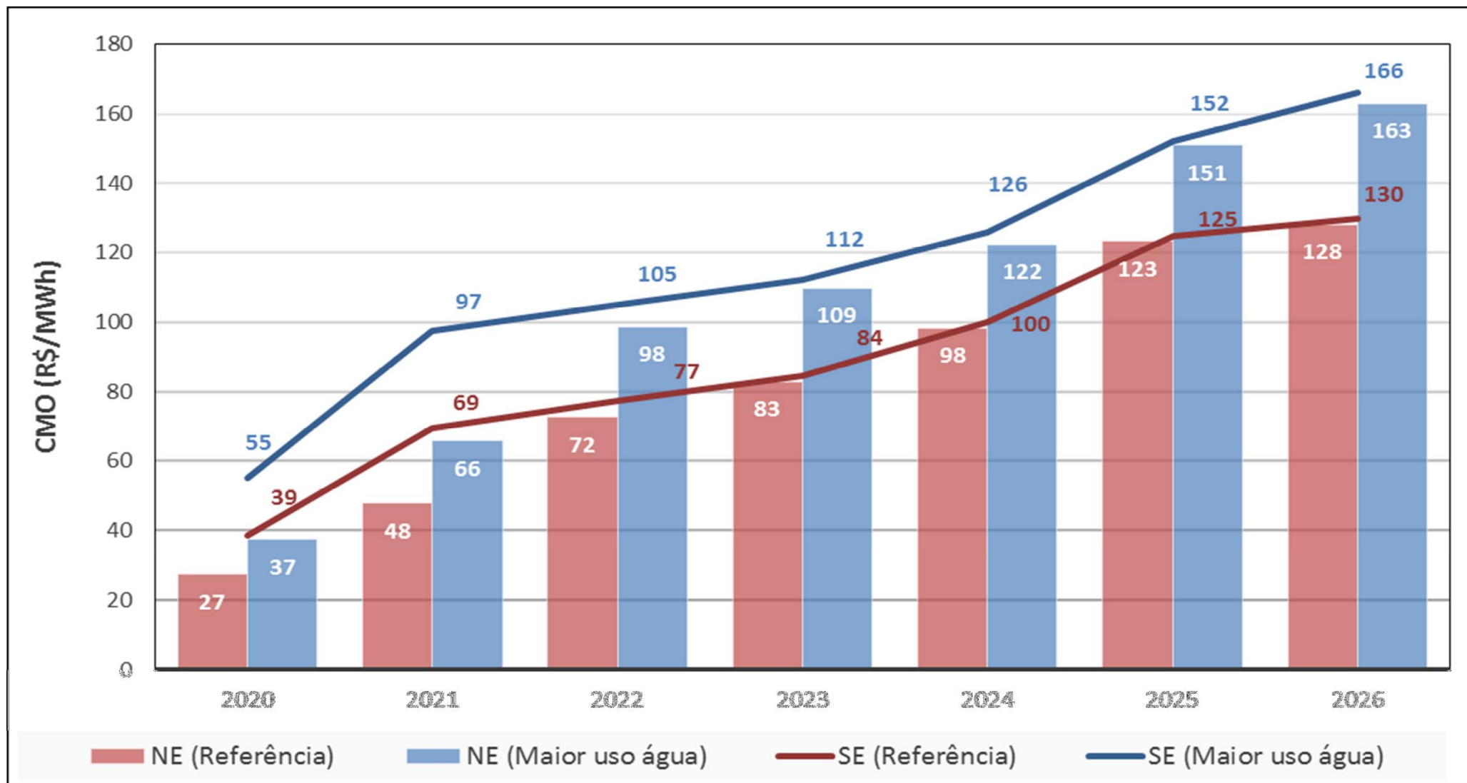
Gráfico 43. CMO para os Cenários de Mercado de Referência e de Maior Uso da Água – Regiões Sudeste e Nordeste
