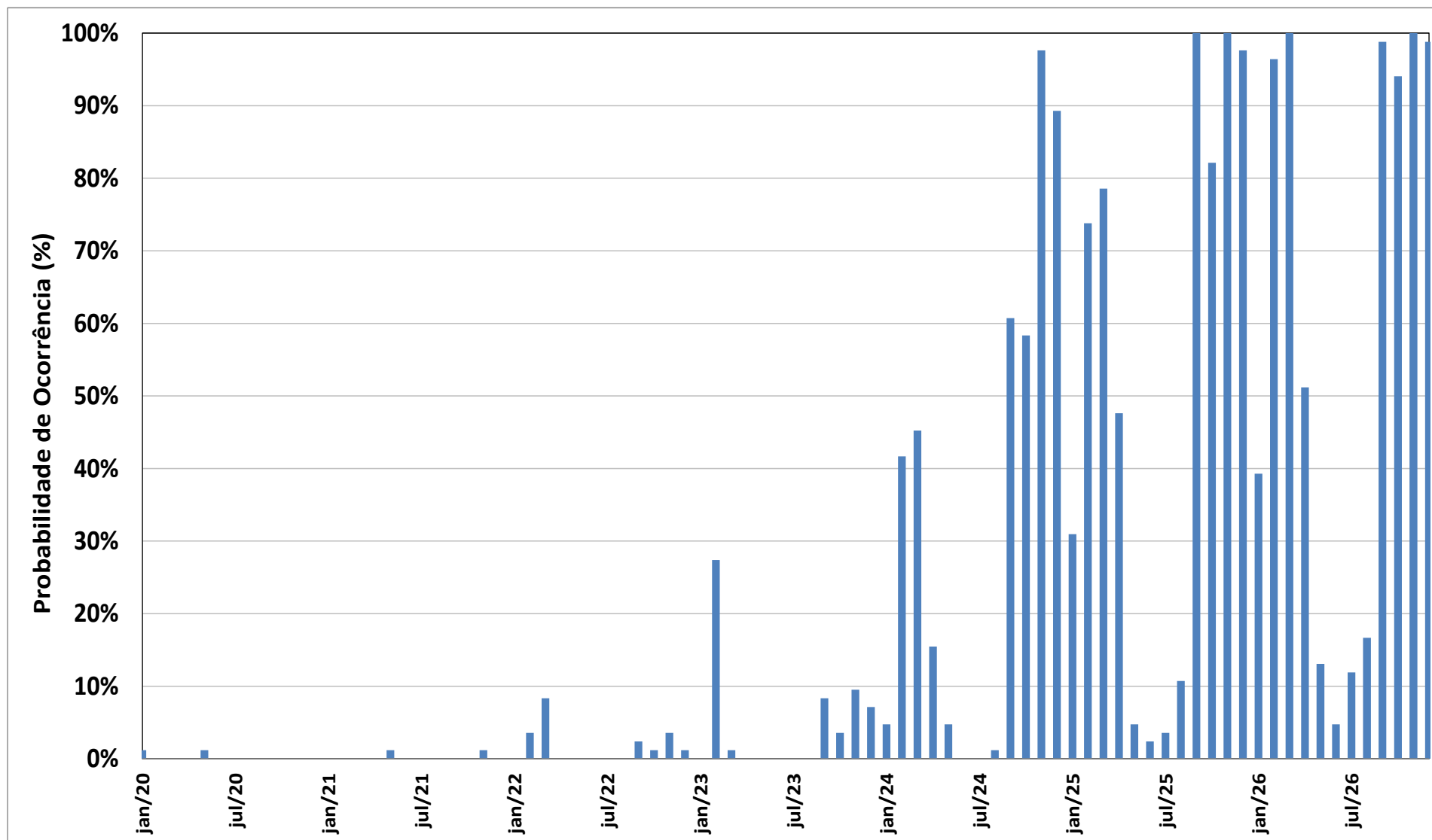
Gráfico 29. Risco de Déficit de Potência na Expansão para o Atendimento apenas à Carga de Energia
