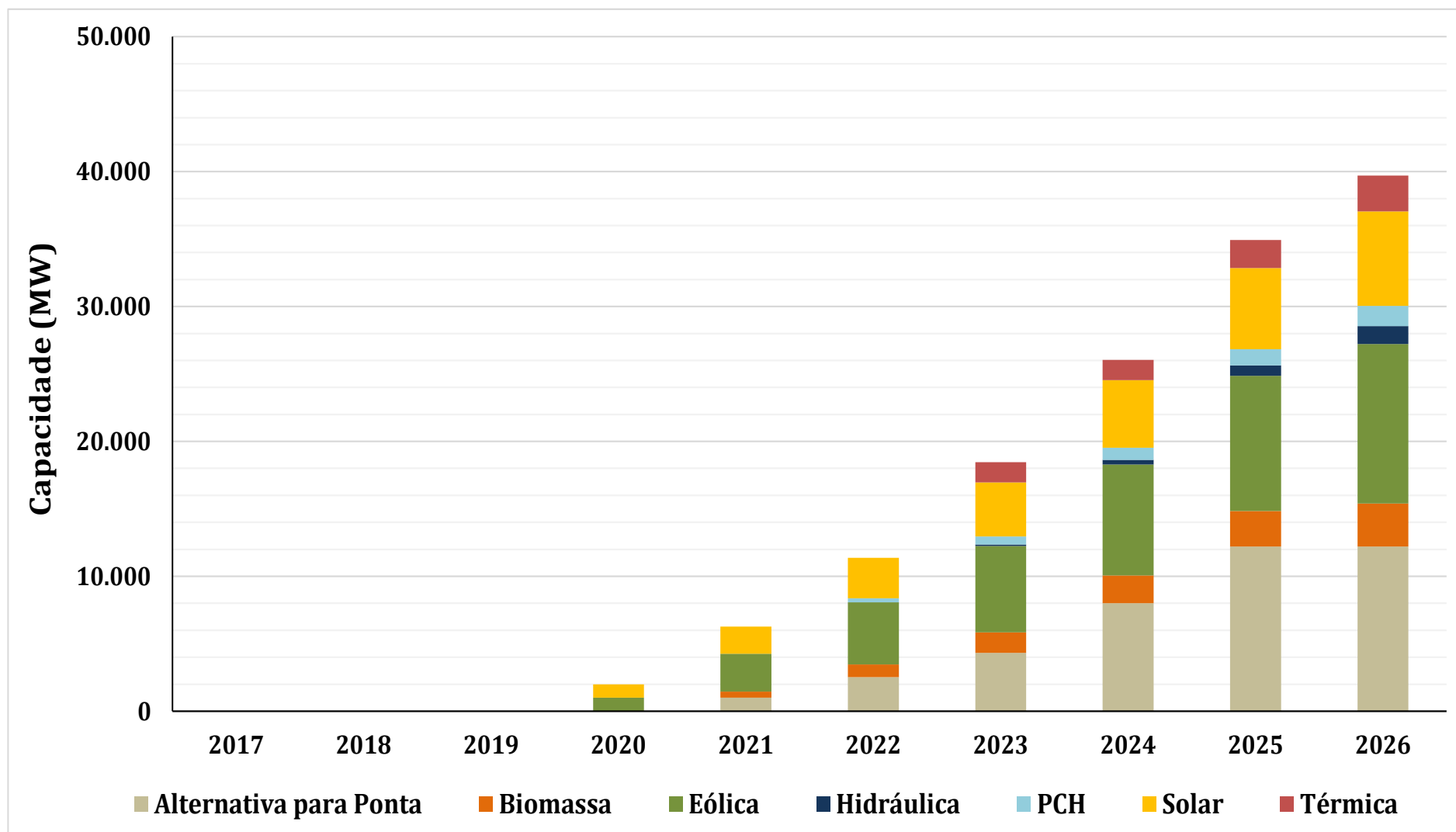
Gráfico 30. Expansão Indicativa de Referência
