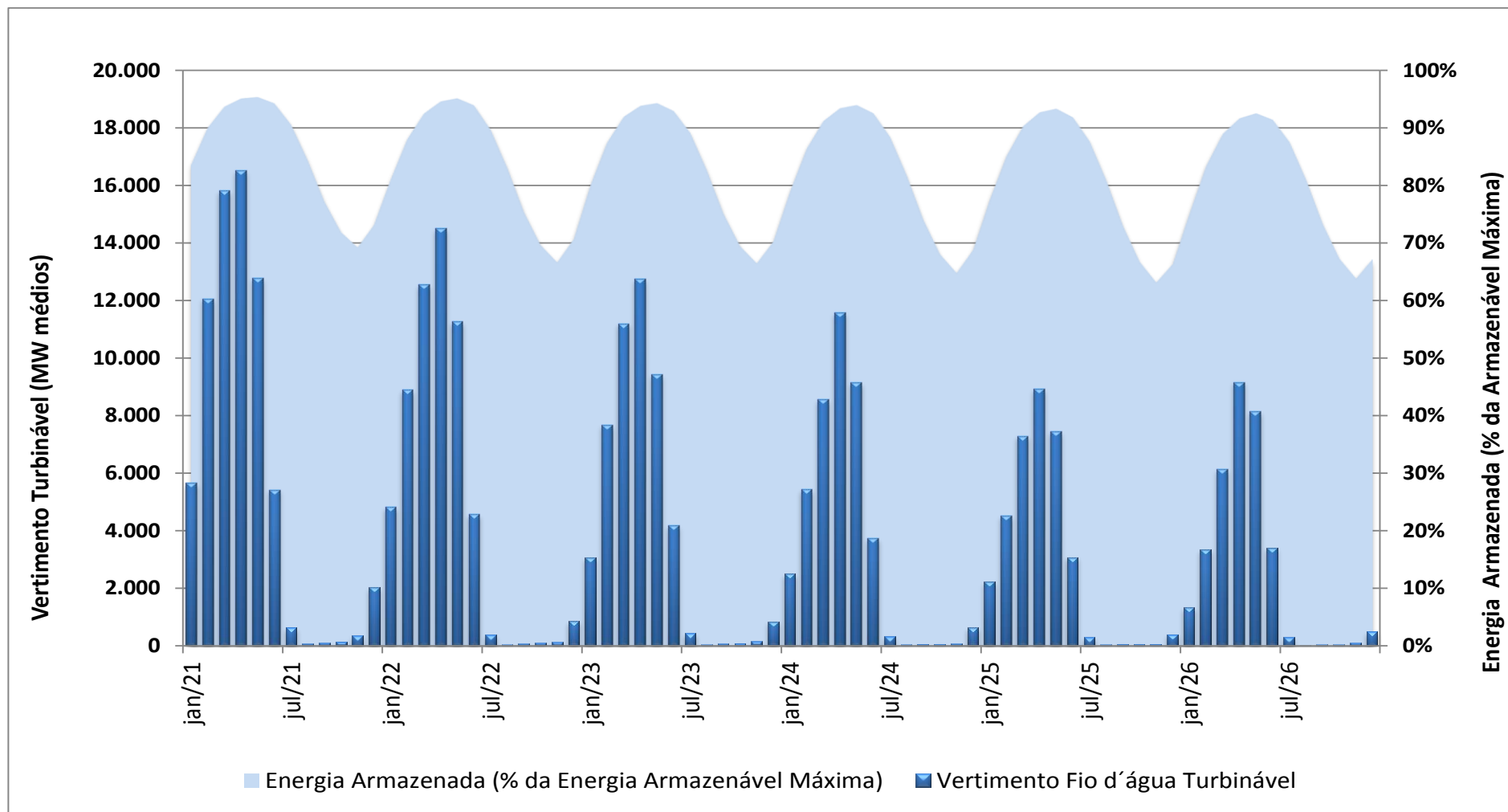
Gráfico 33. Vertimento Turbinável e Armazenamento
