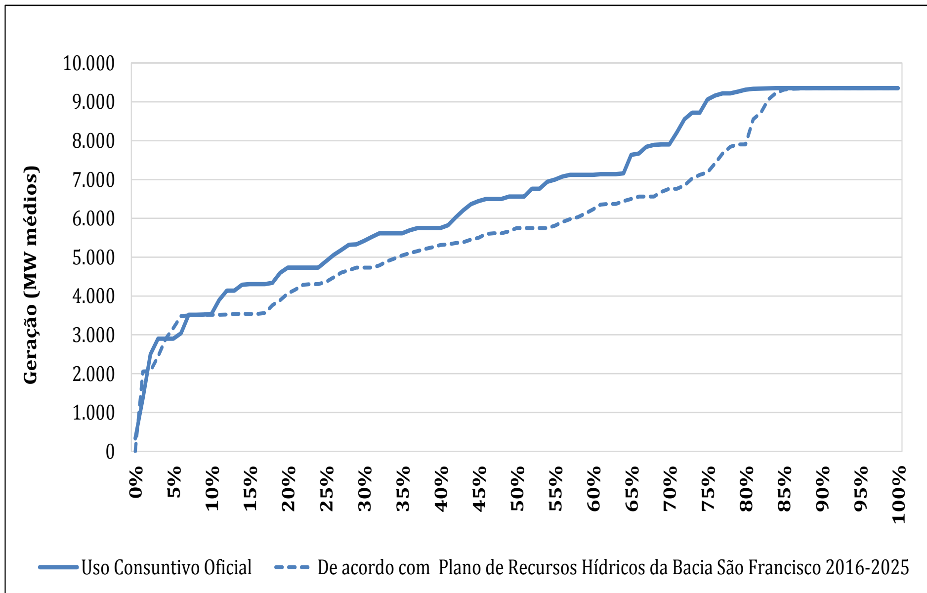
Gráfico 42. Permanência da Geração Hidráulica no Nordeste em 2020
