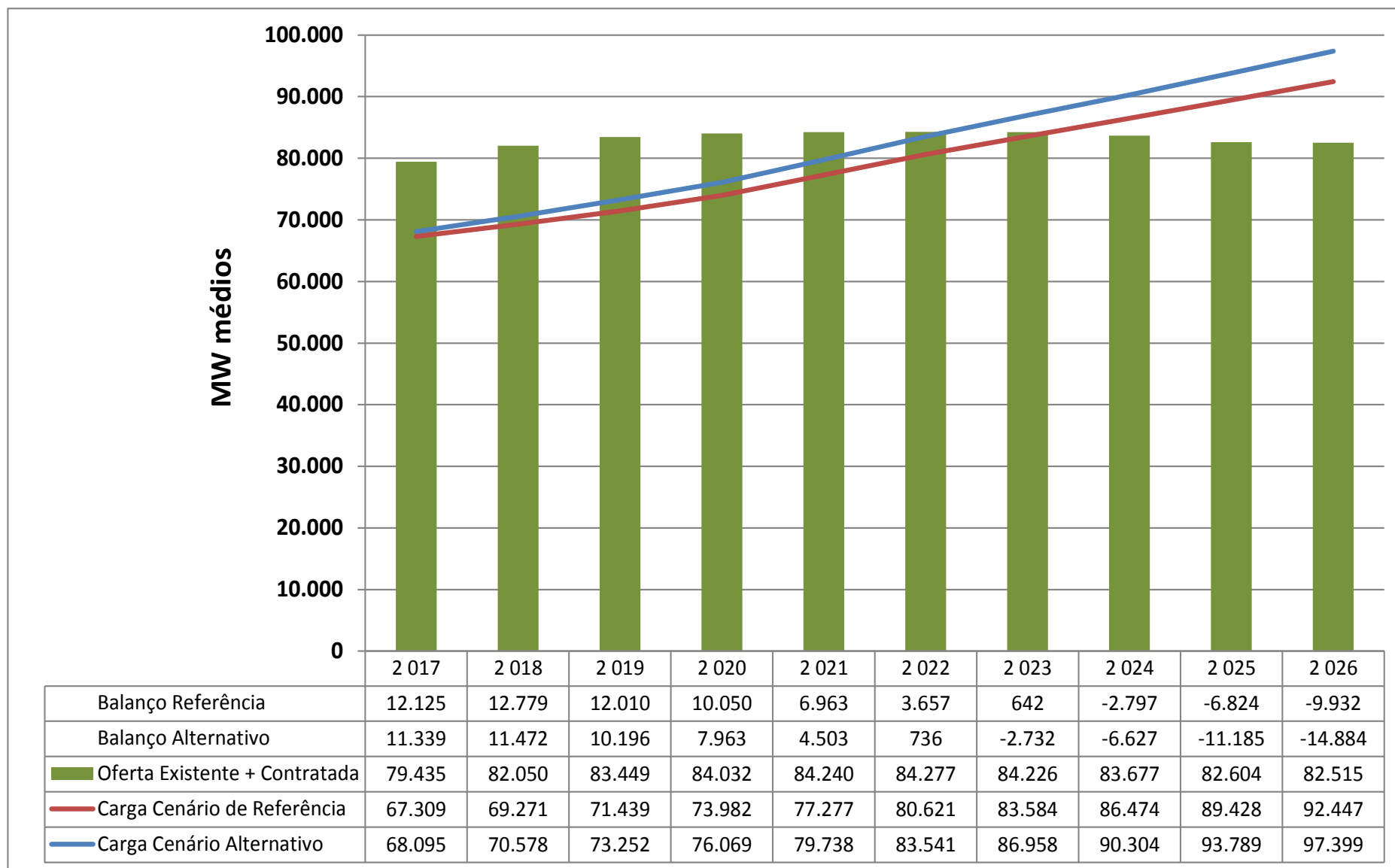
Gráfico 38. Comparação entre as projeções de demanda
