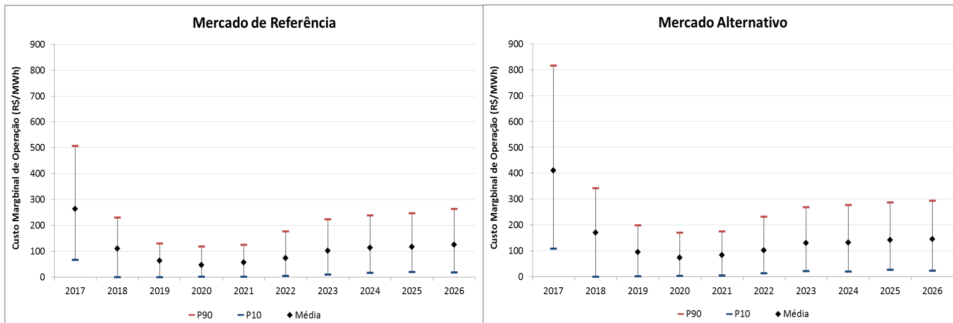
Gráfico 47. Expansão de Referência – Dispersão do Custo Marginal de Operação
