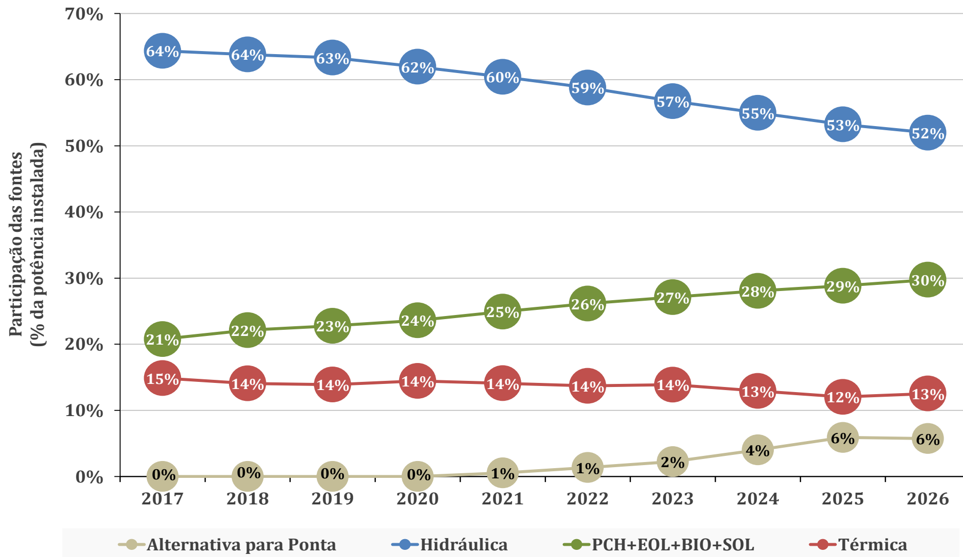
Gráfico 31. Participação das Fontes
