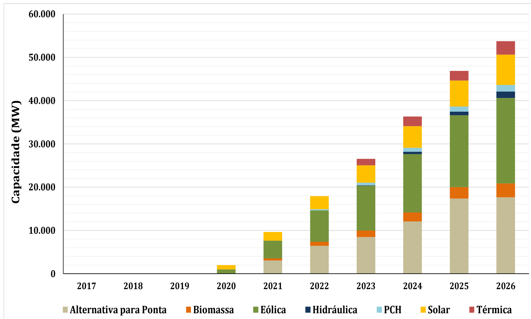
Gráfico 39. Expansão Indicativa - Mercado Alternativo
