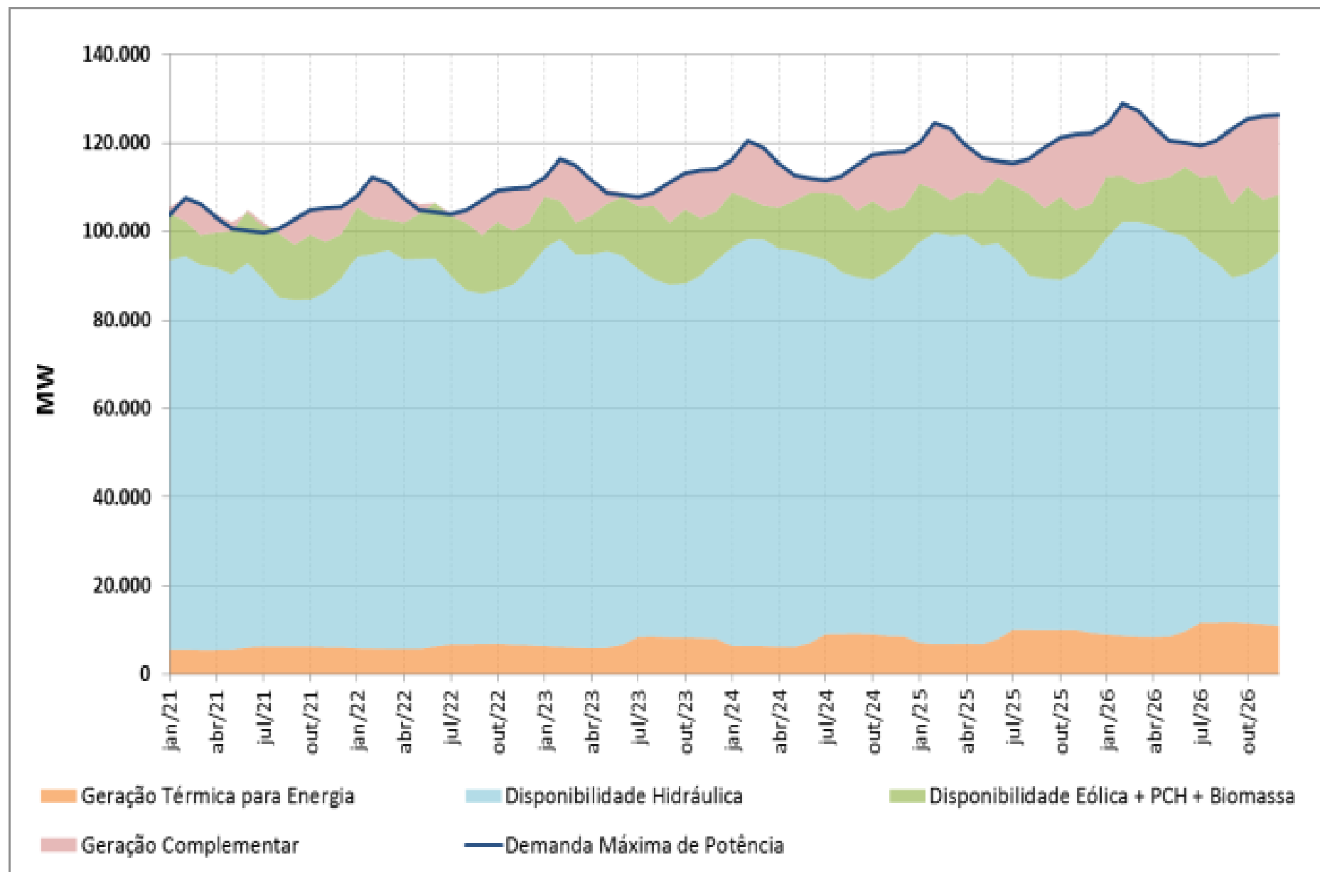
Gráfico 34. Atendimento à Demanda Máxima do SIN
