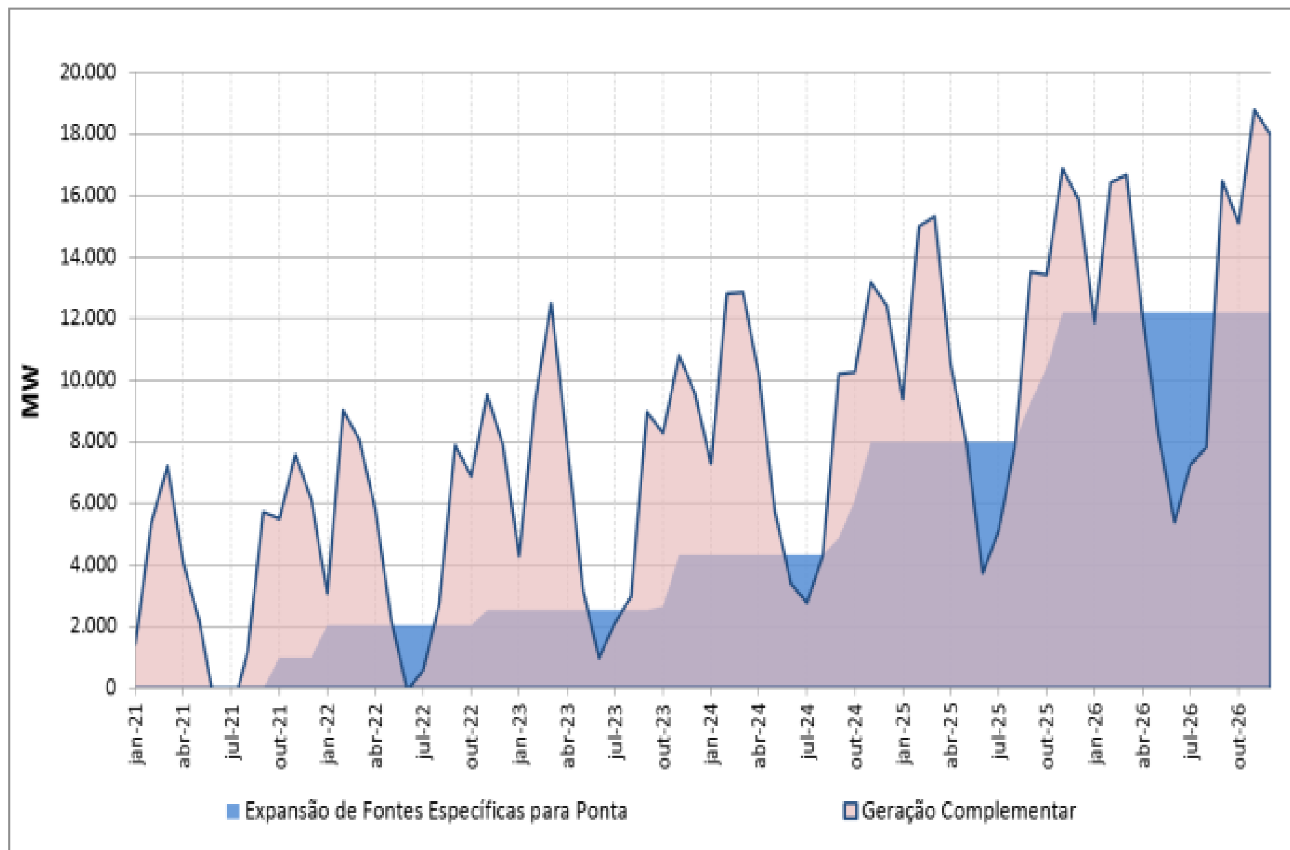
Gráfico 35. Geração Complementar x Alternativa de Ponta
