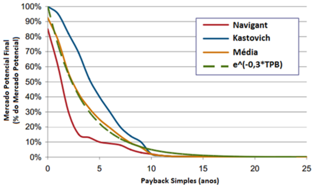
Figura 8 – Mercado Potencial Final vs. Payback – Fonte: KONZEN, 2014.
