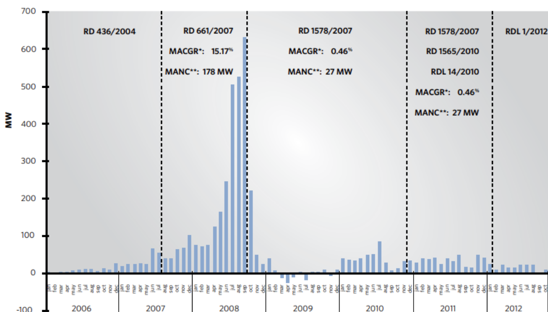
Figura 11 – Instalações mensais de sistemas fotovoltaicos na Espanha. Fonte: DEL RÍO e MIR-ARTIGUES, 2014
