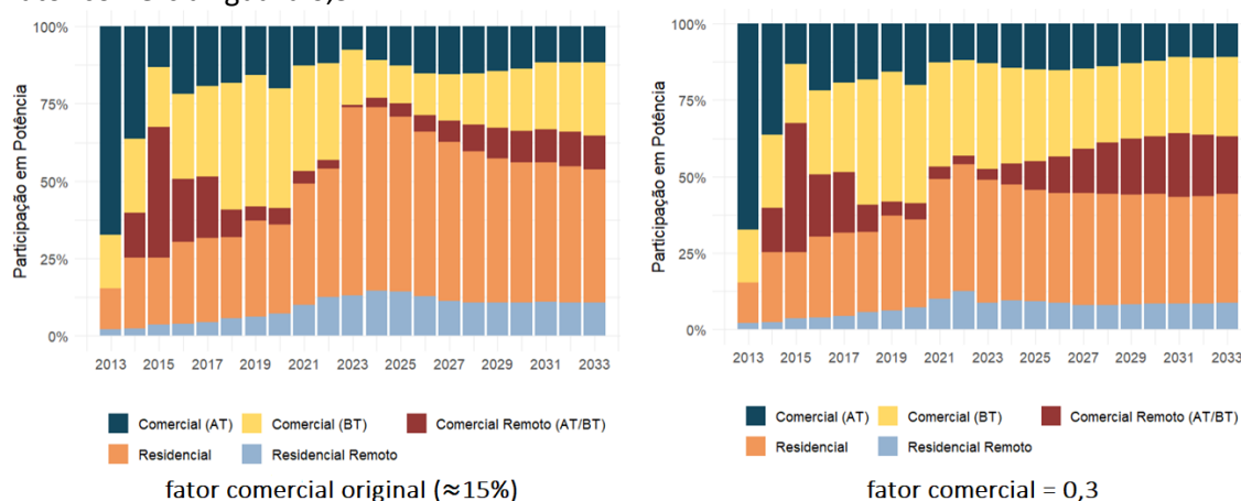
Figura 6 - Potência instalada anual por segmento com diferentes fatores comerciais
