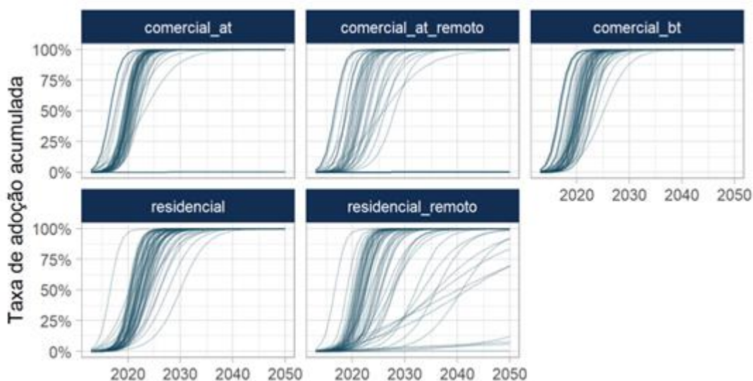
Figura 9 - Exemplo de curvas de adoção
