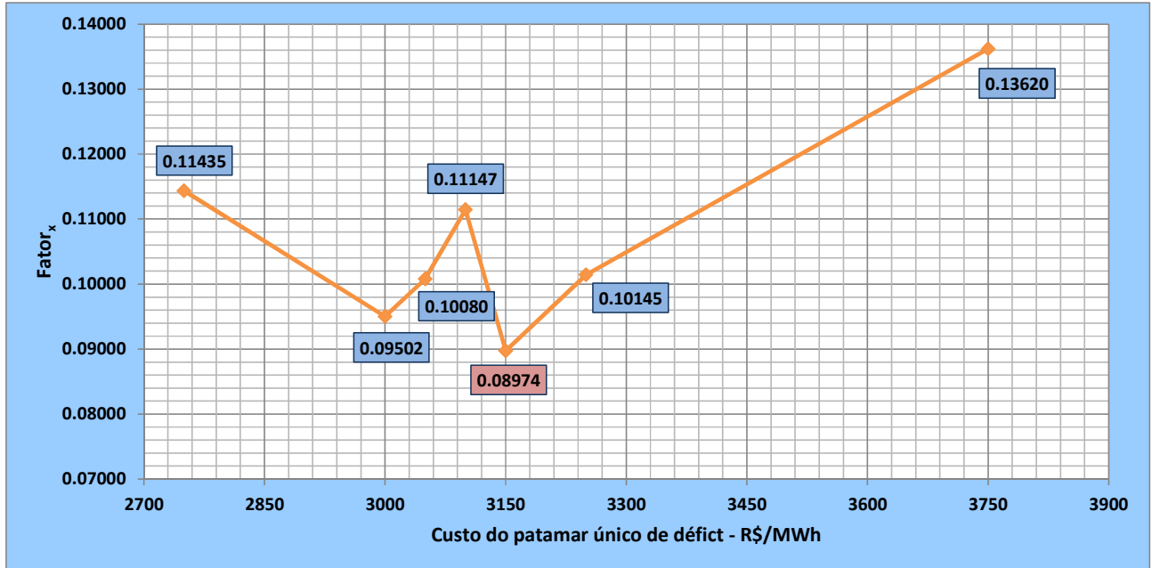
Gráfico 3 – Processo Iterativo para Determinação em Patamar Único
