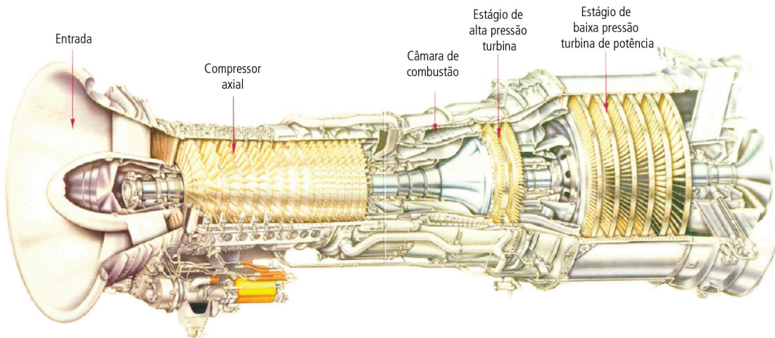
Figura 4 – Turbina aeroderivativa
