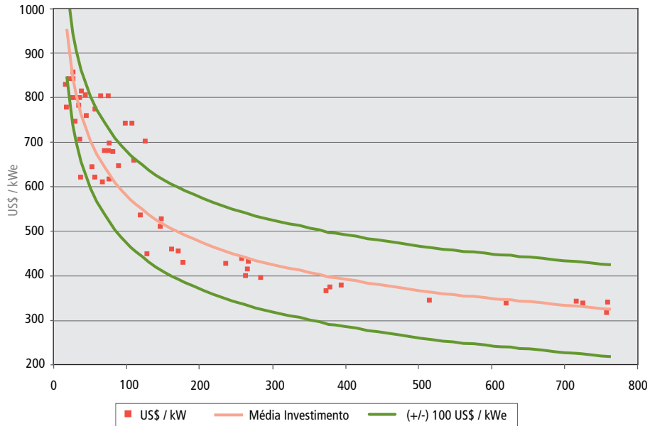
Figura 7 – Custo específico de ciclo combinado
