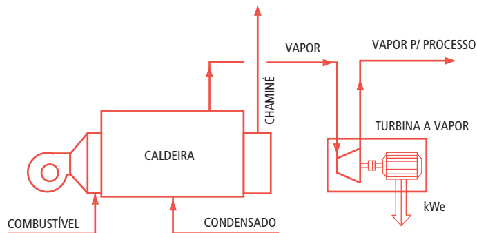
Figura 9 – Configuração bottoming
