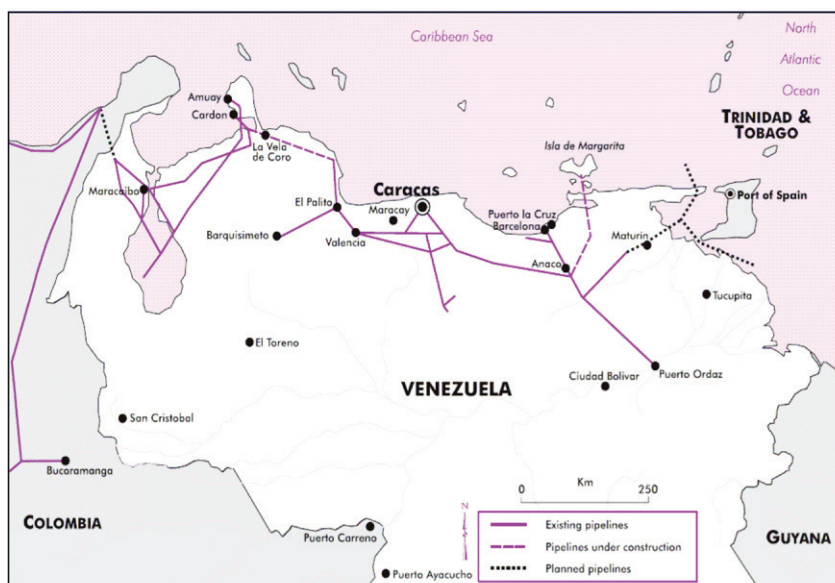
Figura 24 – Infra-estrutura de transporte de gás natural na Venezuela em 2002
