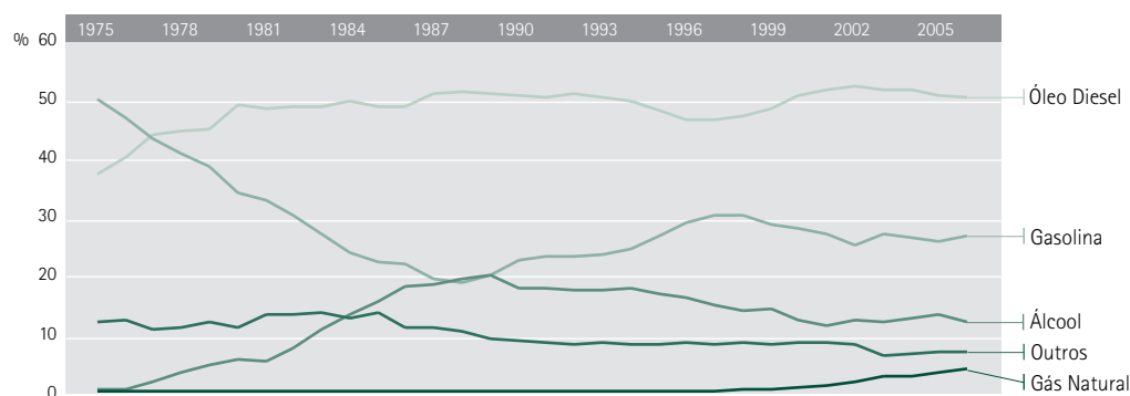
■ Gráfico 3.4 | Estrutura do Consumo no Setor de Transportes
