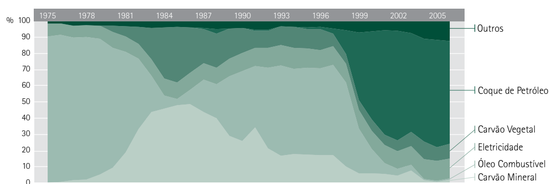
■ Gráfico 3.6 | Estrutura do Consumo no Setor de Cimento
