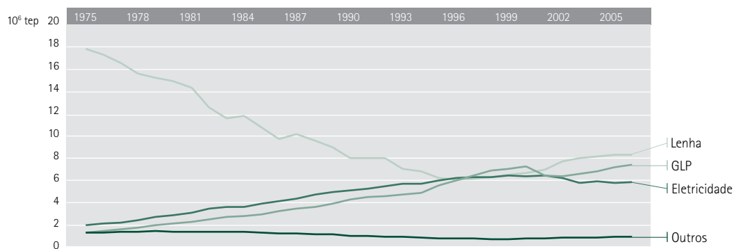
■ Gráfico 3.2 | Consumo Final no Setor Residencial
