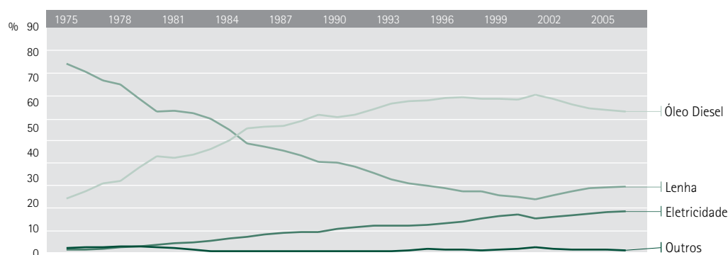
■ Gráfico 3.3 | Estrutura do Consumo no Setor Agropecuário
