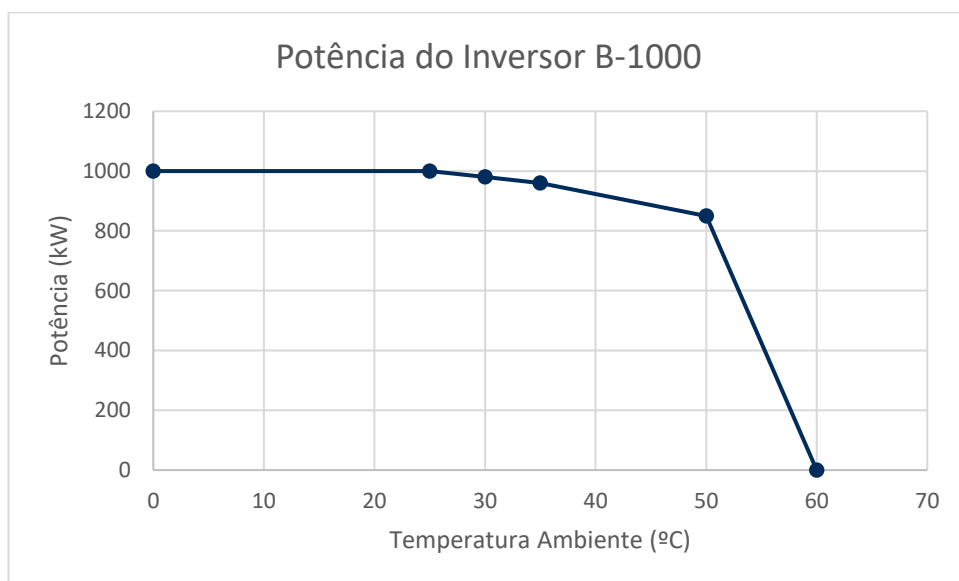
Figura 1 – Comportamento do inversor fictício B-1000 com a temperatura ambiente
