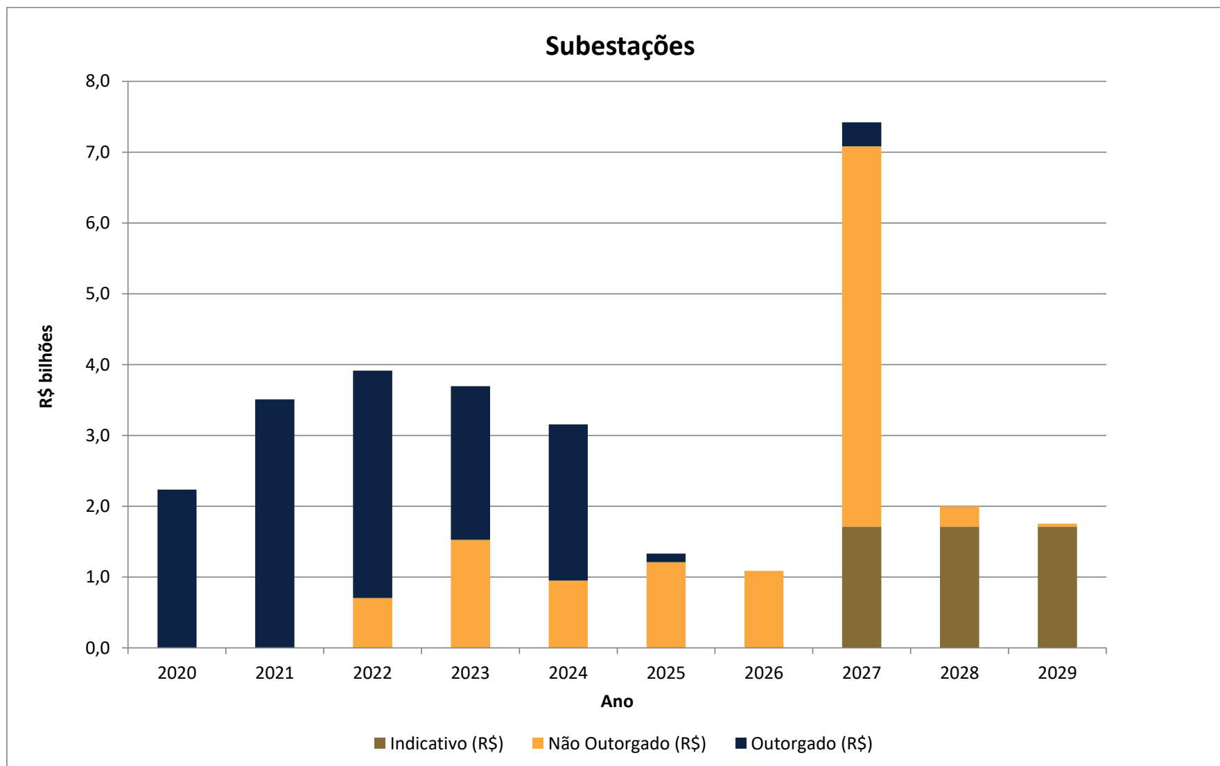
Gráfico 4-5. Investimento em subestações por ano
