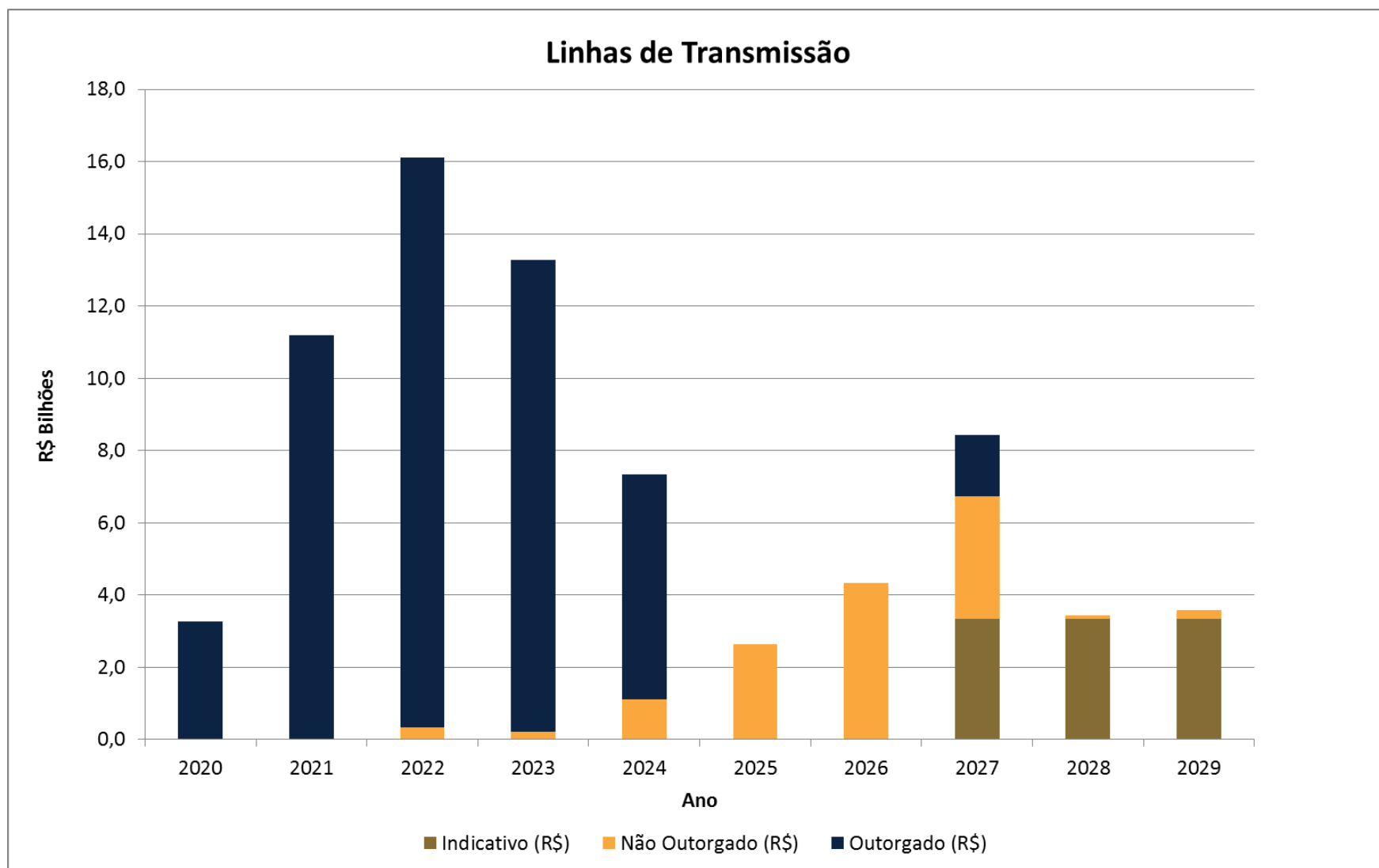
Gráfico 4-4. - Investimento em linhas de transmissão por ano
