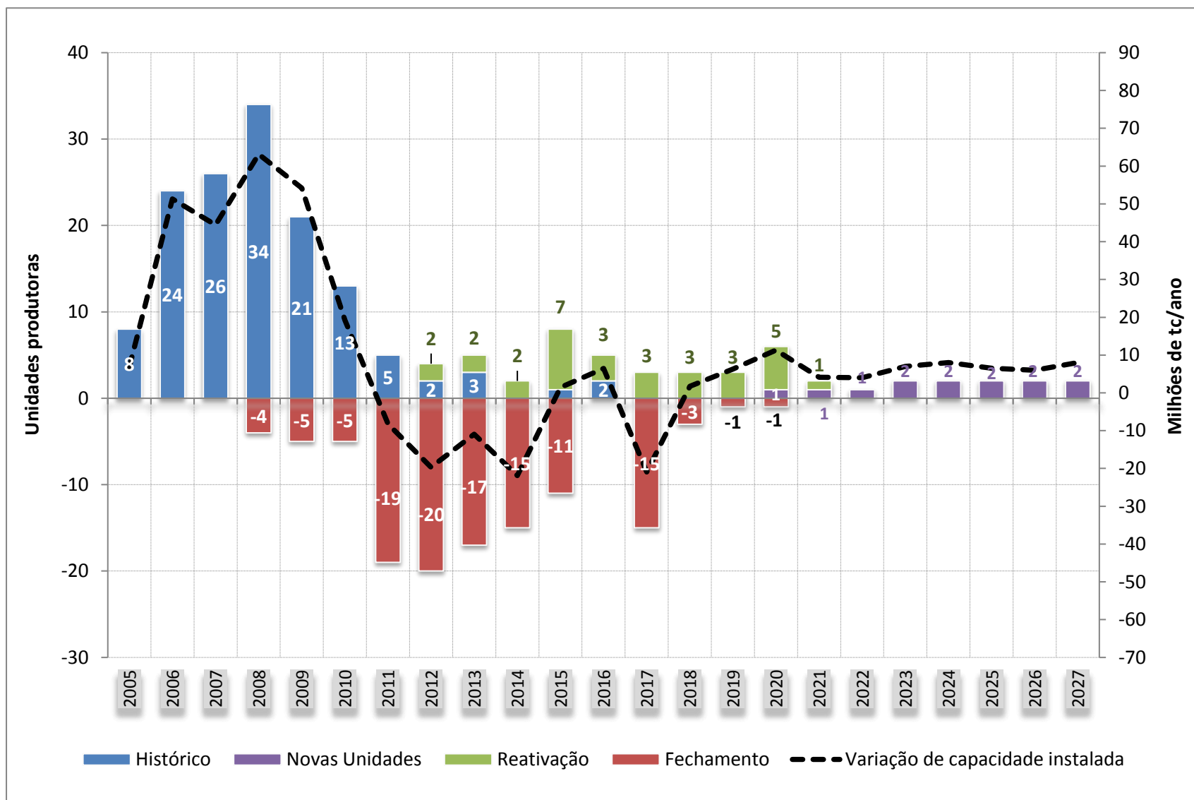
Gráfico 8-1. Fluxo de unidades produtoras de cana-de-açúcar e variação de capacidade instalada
