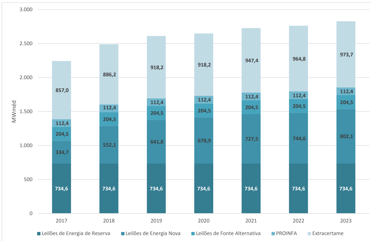
Gráfico 8-6. - Energia contratada e extra certame das usinas vencedoras nos Leilões de Energia
