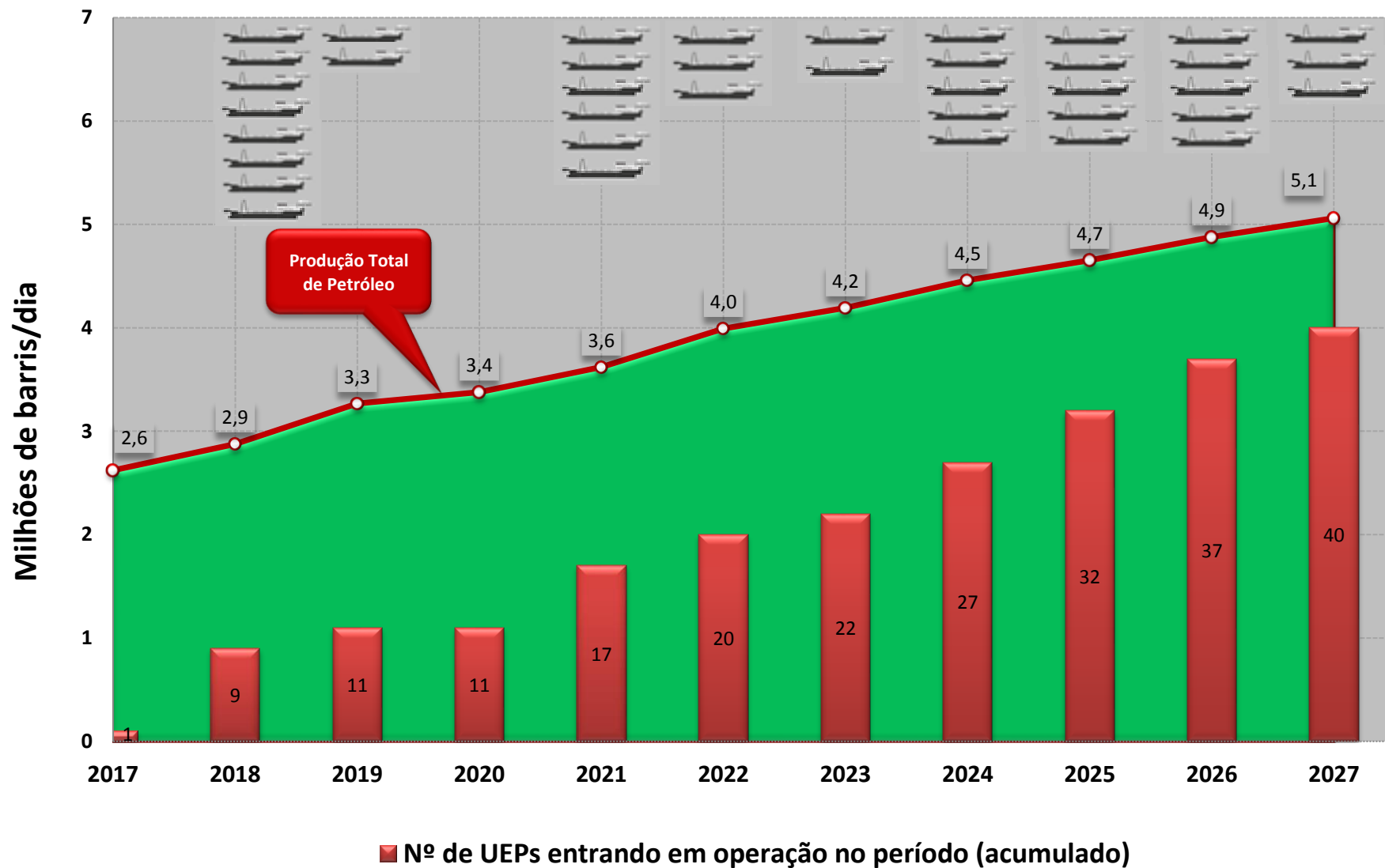
Gráfico 5-12. - Previsão de entrada em operação de novas UEP
