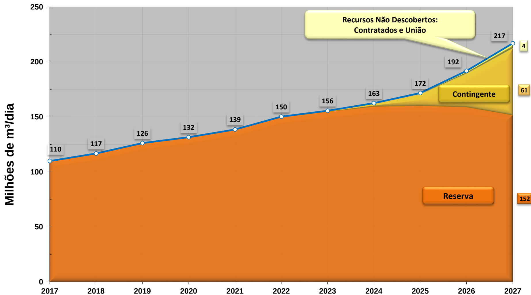
Gráfico 5-2. Previsão de produção bruta diária de gás natural nacional
