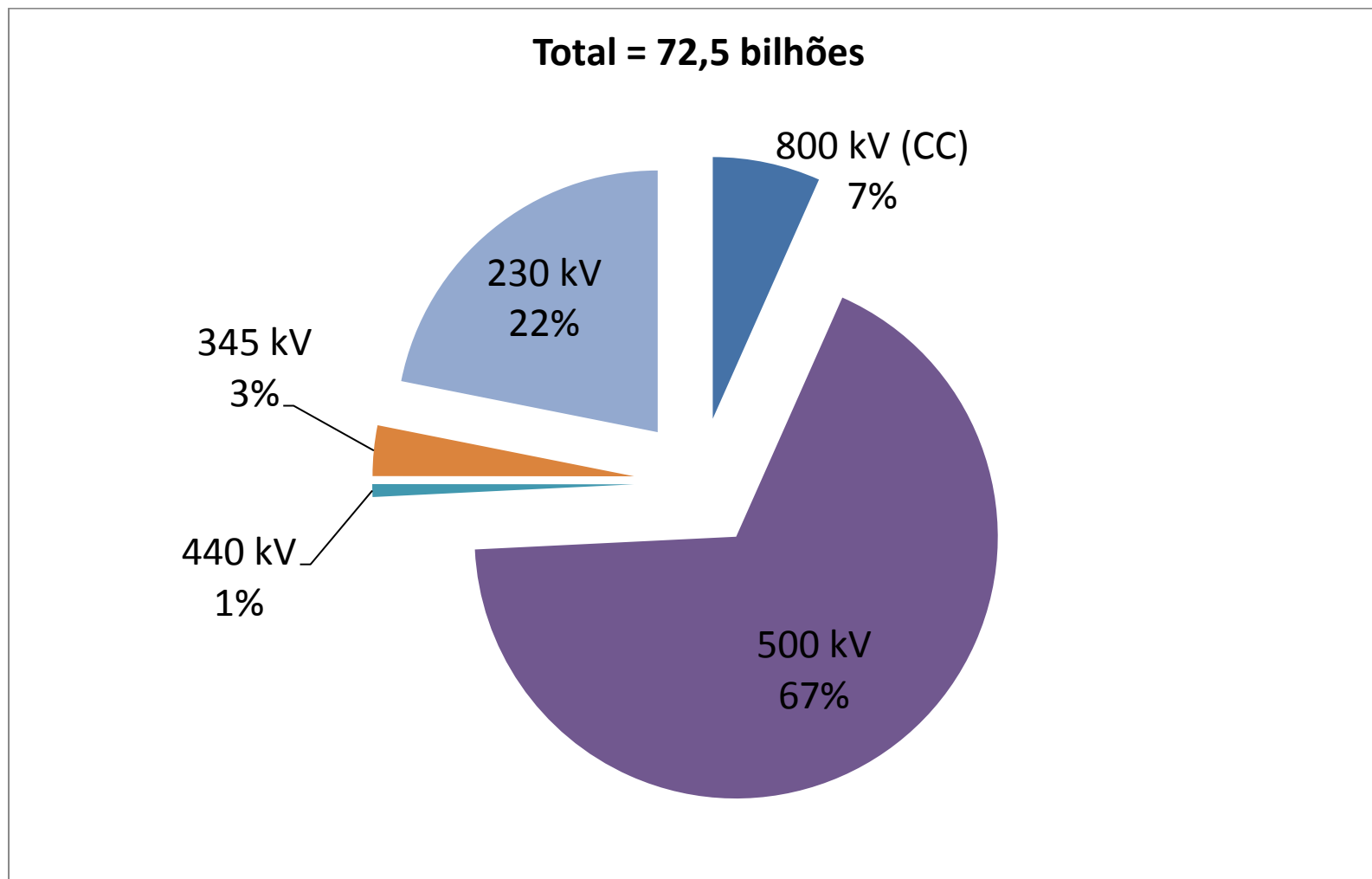
Gráfico 4-2. Investimento total em linhas de transmissão, por nível de tensão
