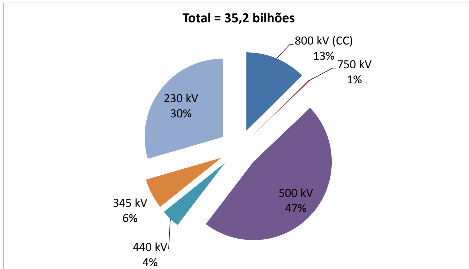
Gráfico 4-3. - Investimento total em subestações, por nível de tensão
