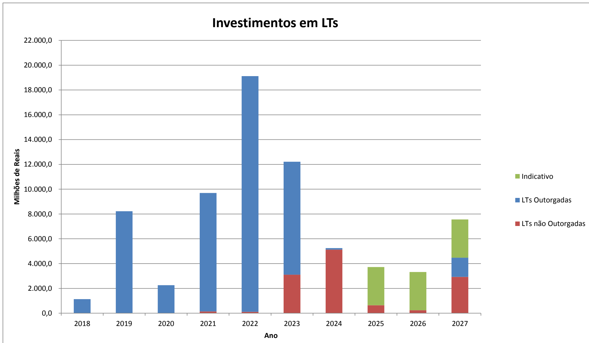
Gráfico 4-4. Investimento em linhas de transmissão
