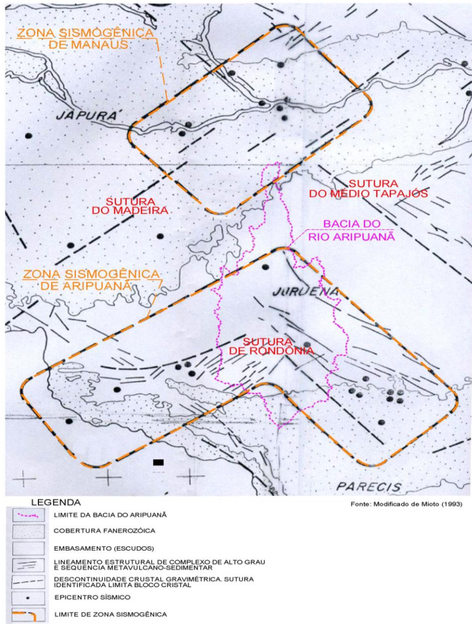
Figura 2.3.2. – Localização da bacia do rio Aripuanã nas zonas sismogênicas, definidas por Miotto (1993).
